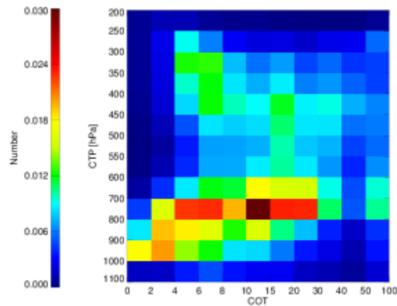
MODIS
